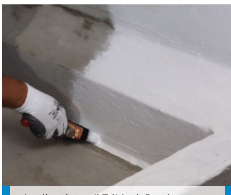
Applicazione di Triblock P nel raccordo tra platea e muro di elevazione
