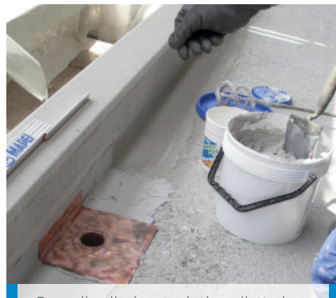
Posa di collarino e relativa piletta in rame
