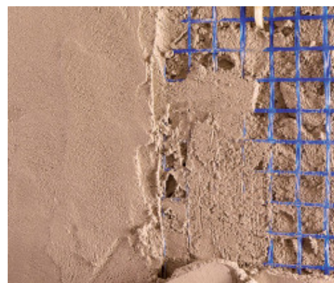
Applicazione del secondo strato di MapeWall Intonaca & Rinforza 10
