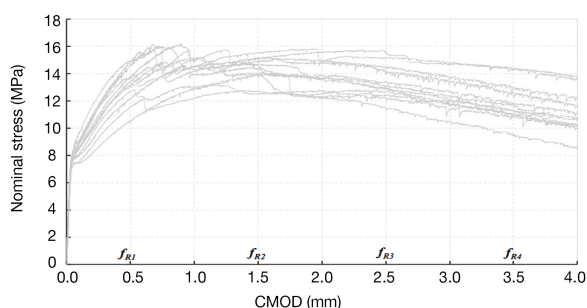
Resistenza a flessione residua in accordo alla norma EN 14651
