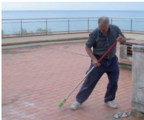
Pulizia del supporto prima dell'applicazione di Aquaflex Roof
